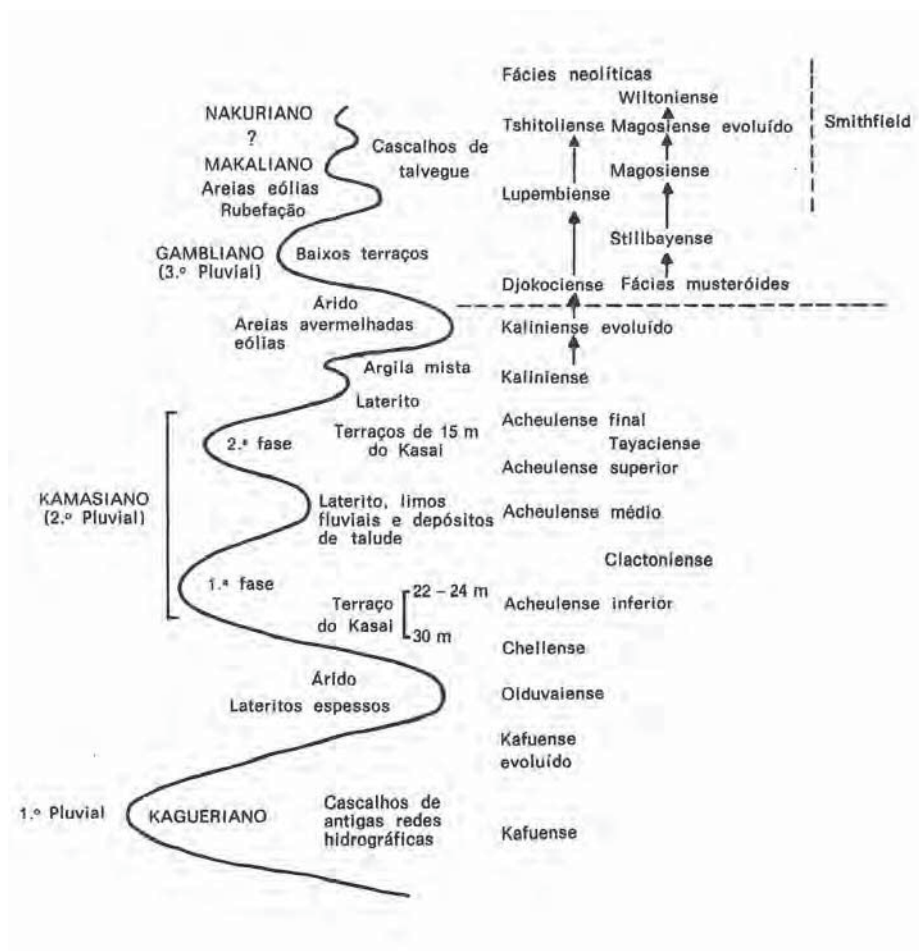
FIGURA 21.1 Variações climáticas e indústrias pré-históricas da bacia do Zaire (segundo G. Mortelmans, 1952).
