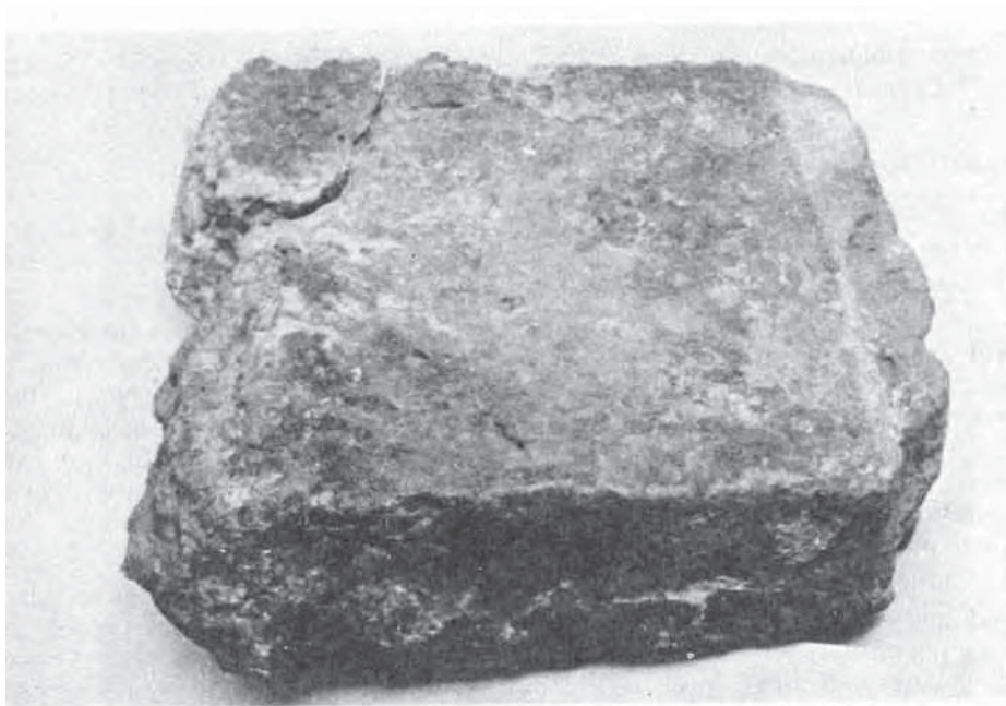
FIGURA 9.3 Bloco de vitrificação mostrando a superfície superior plana, as paredes laterais e uma parte do cadinho ainda aderente ao lado direito.
