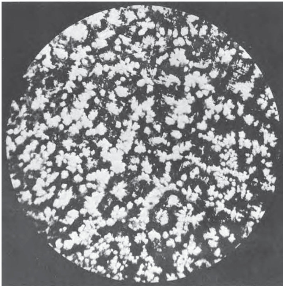
FIGURA 9.1 Microfotografia de uma secção da fateixa de cobre pertencente ao barco de Quéops em Gizé.
