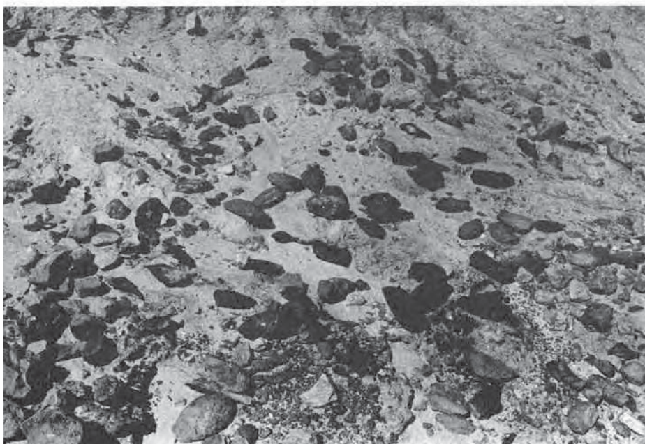
FIGURA 19.6 Isimila, terras altas da Tanzânia meridional. Vista da ravina erodida mostrando as camadas onde foram encontrados utensílios acheulenses (Foto J. E. G. Sutton).
