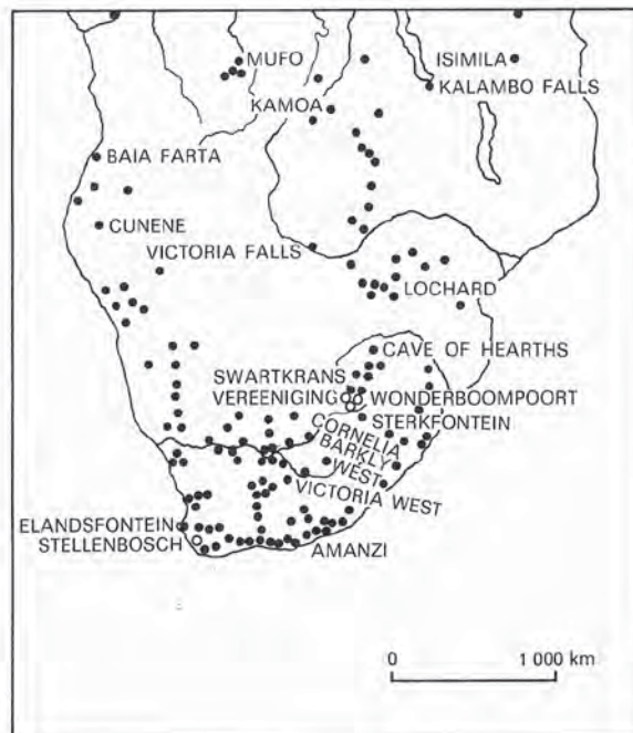
FIGURA 20.3 Principais depósitos de fauna e fósseis humanos do fim do Plioceno (fauna = \Delta ; fósseis humanos = \circ ) ao início do Pleistoceno ( \blacktriangle ; \bullet ) na África austral (Apud CLARK, J. D. The Prehistory of Africa . Londres, Thames and Hudson, 1970. Figs. 9).
